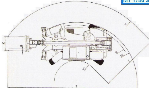
MT 1740 SL TURBO
