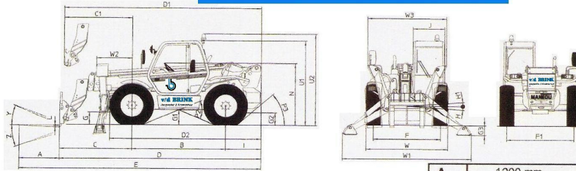
MT 1740 SL TURBO
